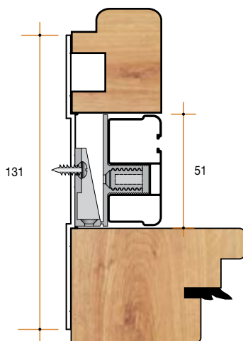
Esempio con guida e compensatore alto
