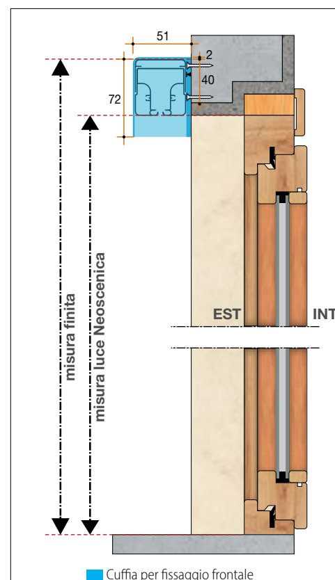
Sezione verticale
