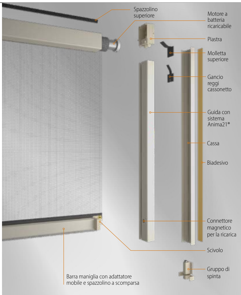
Cassonetto e barra maniglia
