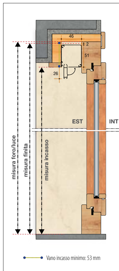
Sezione verticale
