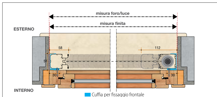
Sezione orizzontale 2 battenti
