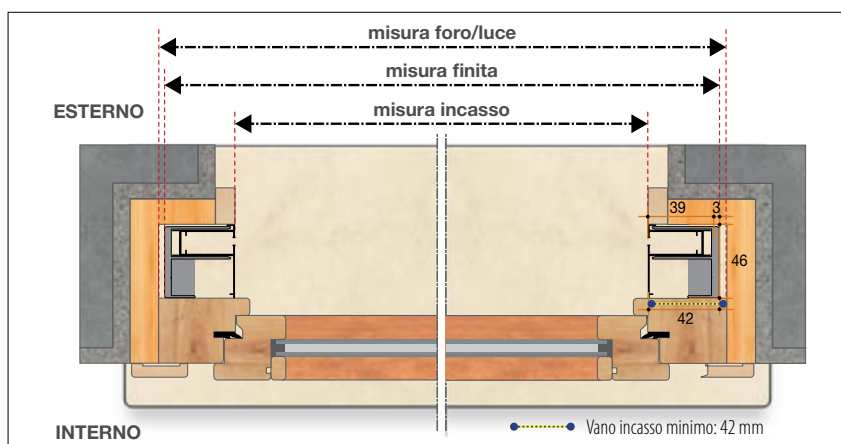
Sezione orizzontale
