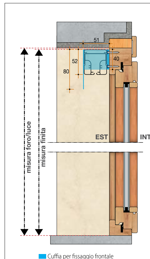
Sezione verticale
