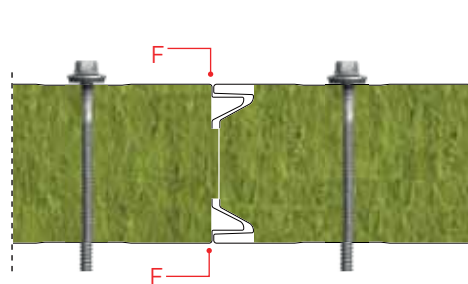
Dettaglio del giunto Tipo 1
