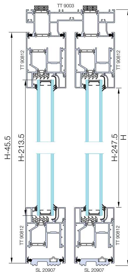
Sez. A-A
