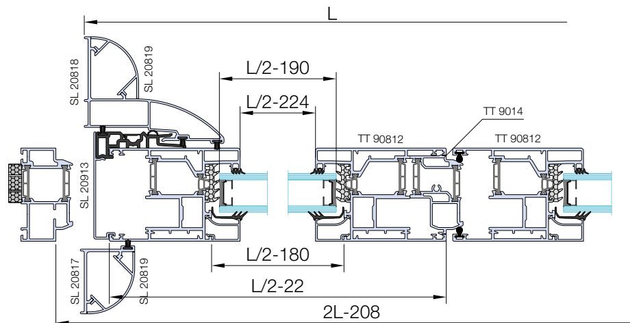
Sez. B-B
