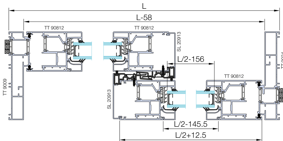
Sez. B-B
