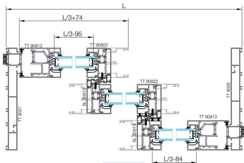
Sez. B-B
