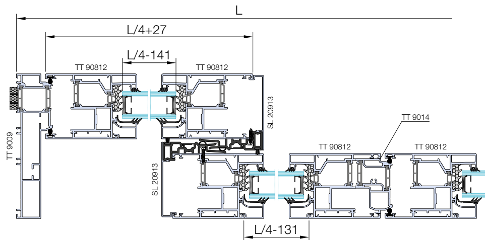
Sez. B-B
