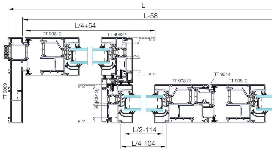
Sez. B-B
