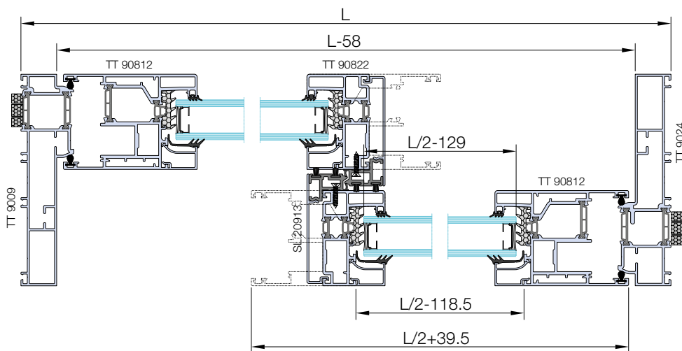
Sez. B-B
