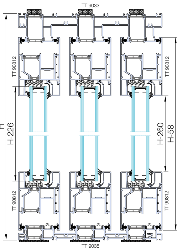
Sez. A-A
