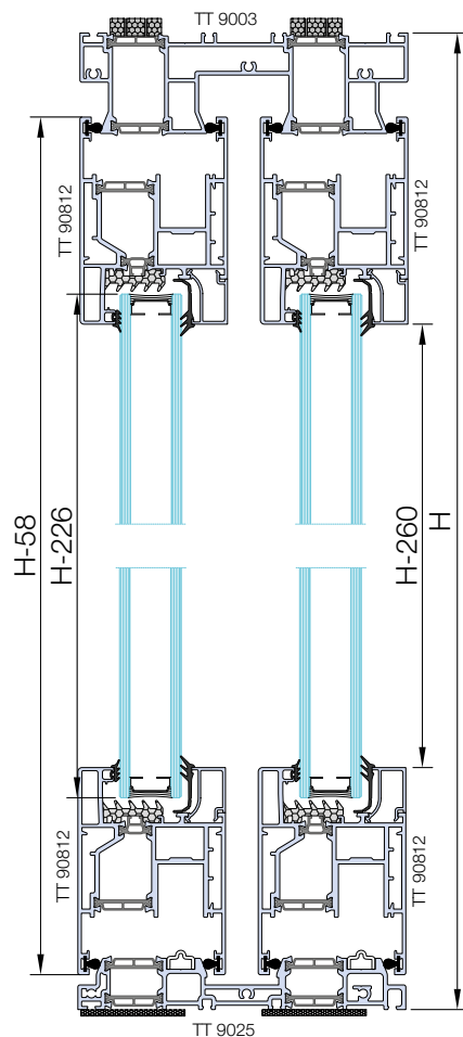
Sez. A-A
