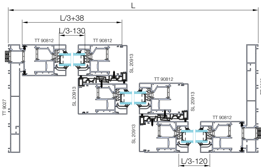
Sez. B-B
