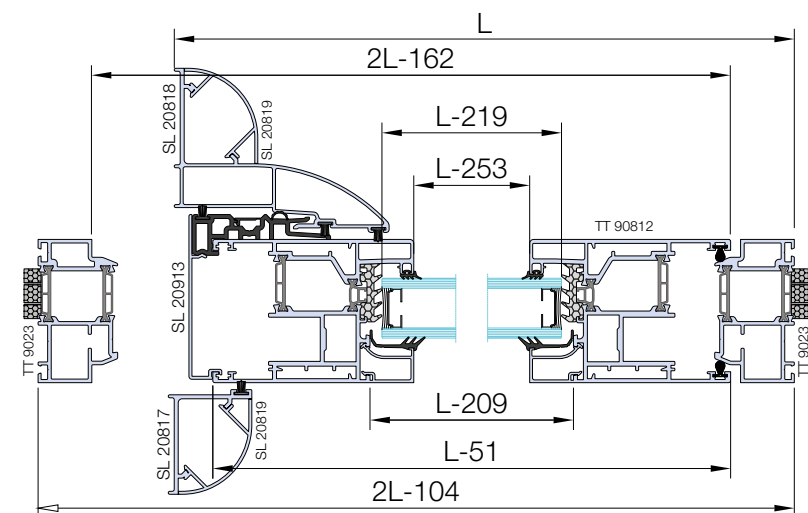
Sez. B-B
