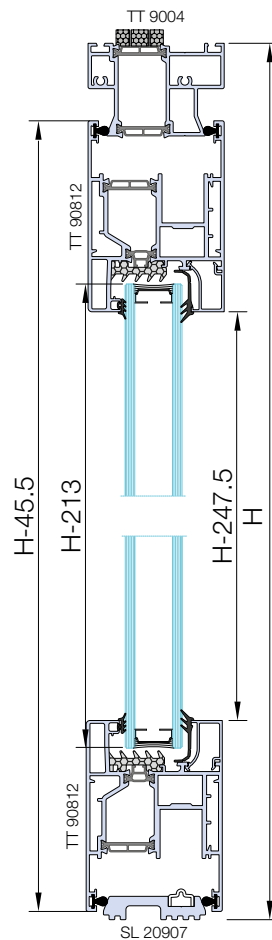
Sez. A-A
